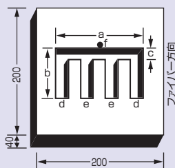
(加工形状・寸法)
